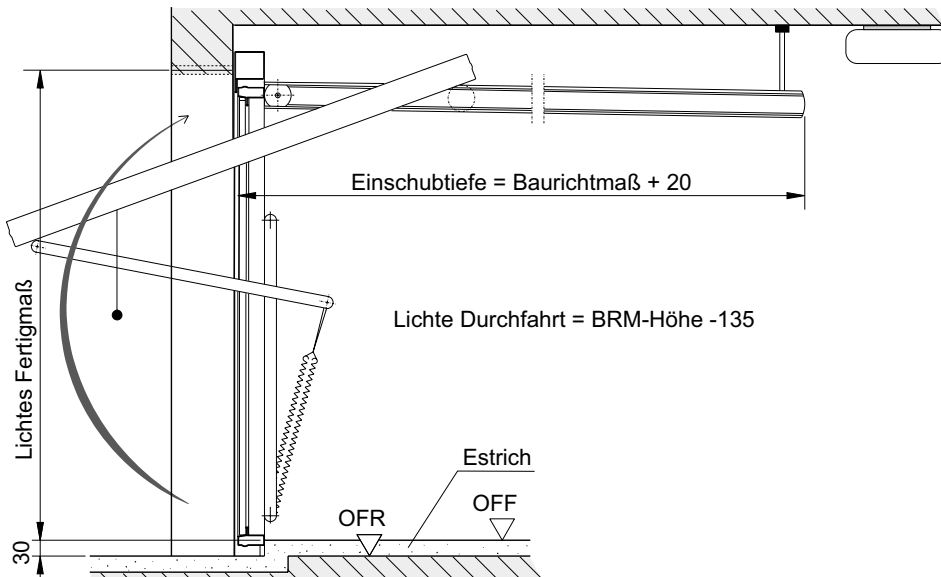
Einschubtiefe
