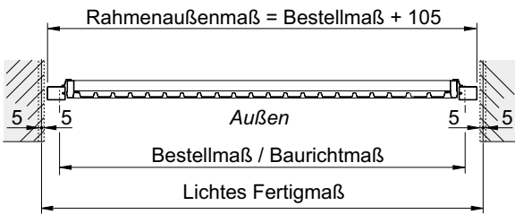
Einbau in der Öffnung
