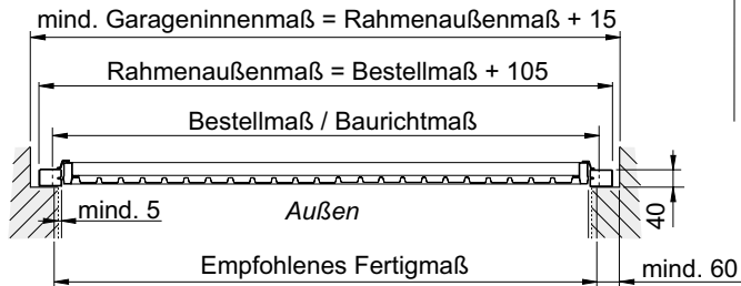
Einbau hinter der Öffnung
